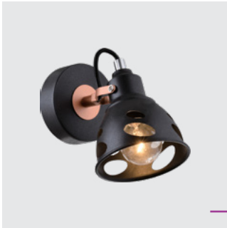
75454 Notos steel-matt black/ red copper 1x E14/40W EAN 8585032233951 E14 ⚡ ⚡
